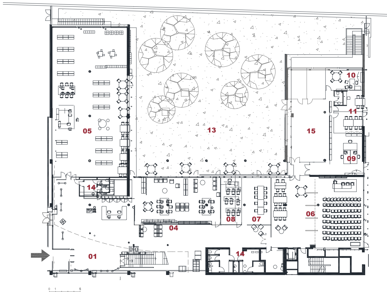
Planta accés
