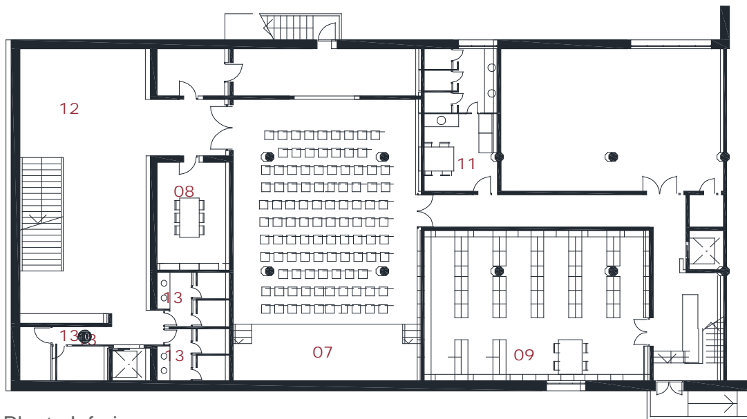
Planta Inferior
