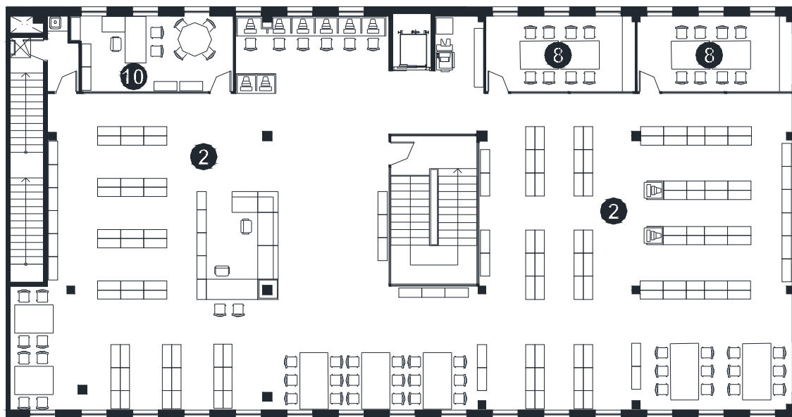
Planta Segona
