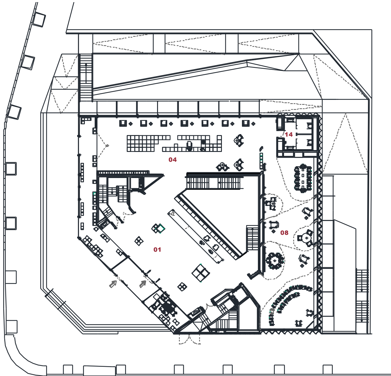
Planta accés 0 1 5
