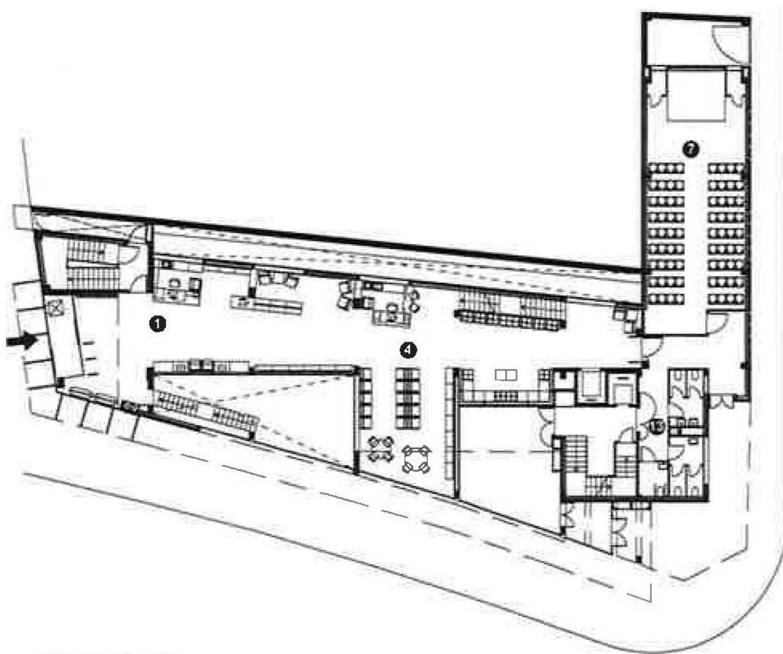
Planta Accés
