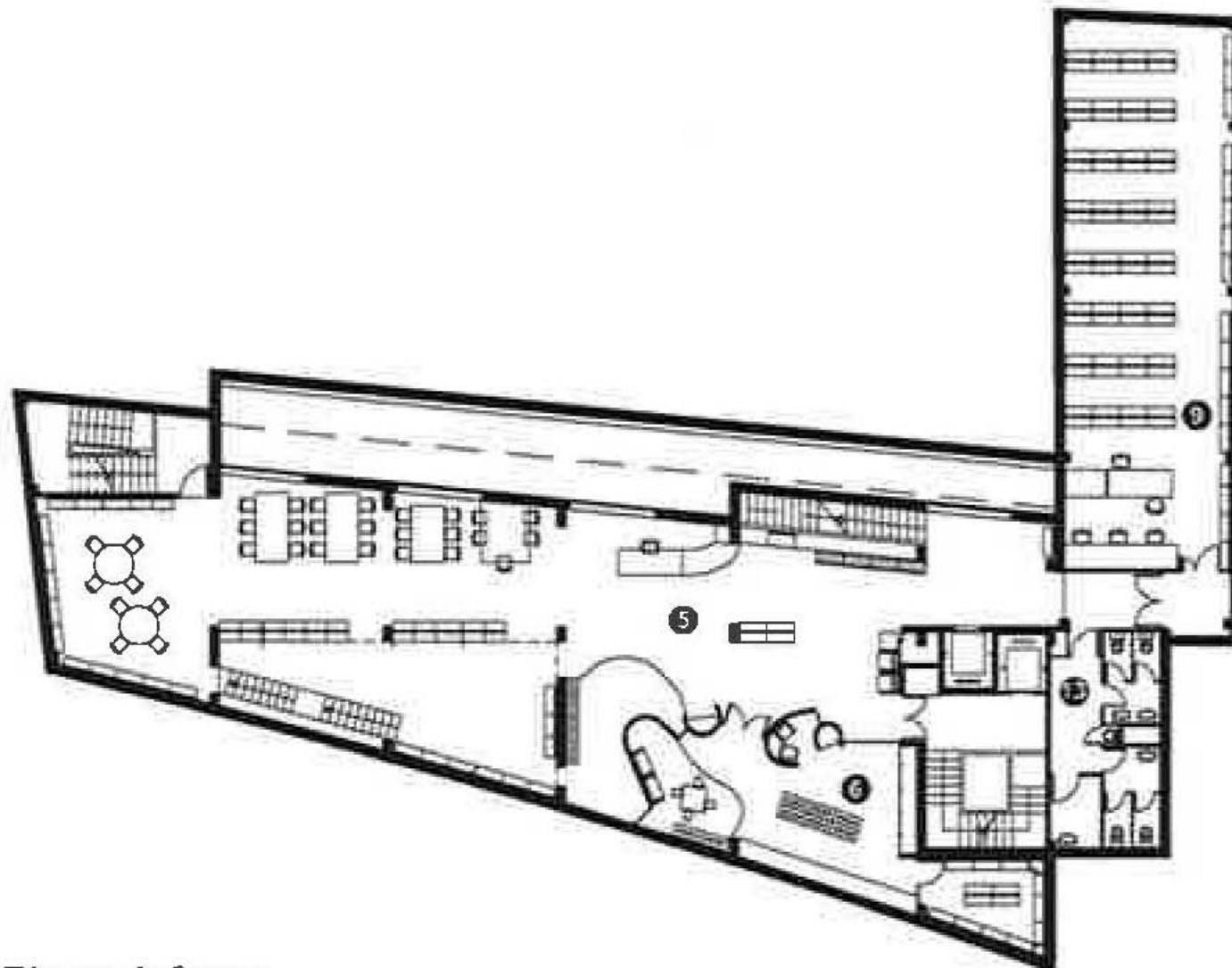
Planta Inferior
