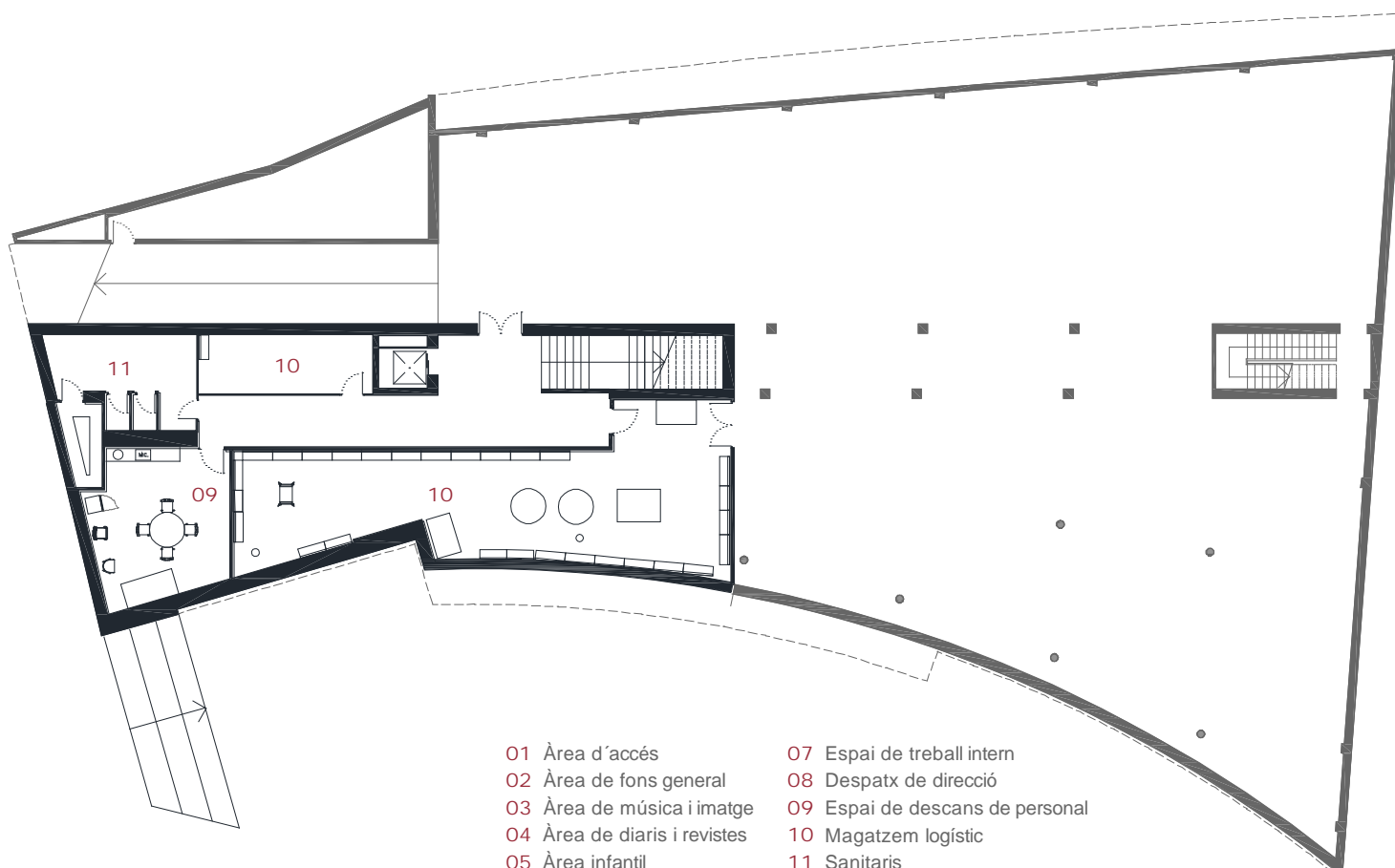
Planta inferior 0 1 5
