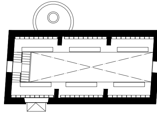
PLANTA ALTELL
